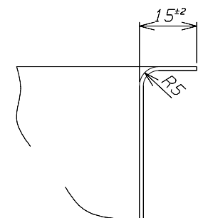
B-B' 断面 S=1/1
