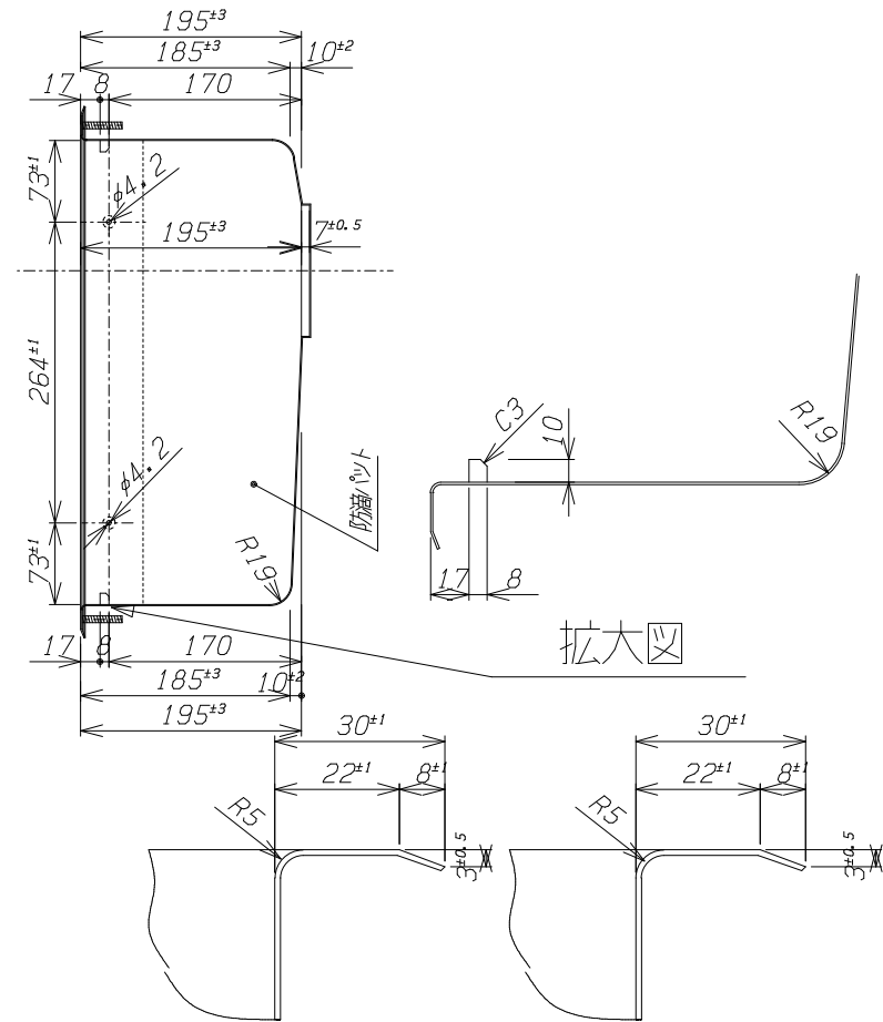
A-A' 断面 S=1/1 B-B' 断面 S=1/1
