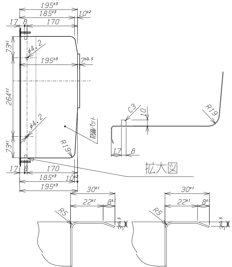
A-A' 断面 S=1/1 B-B' 断面 S=1/1
