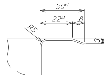
B-B' 断面 S=1/1
