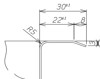
A-A 断面 S=1/1
