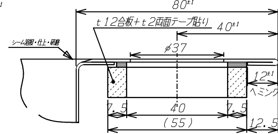
A-A' 断面 S=1/1
