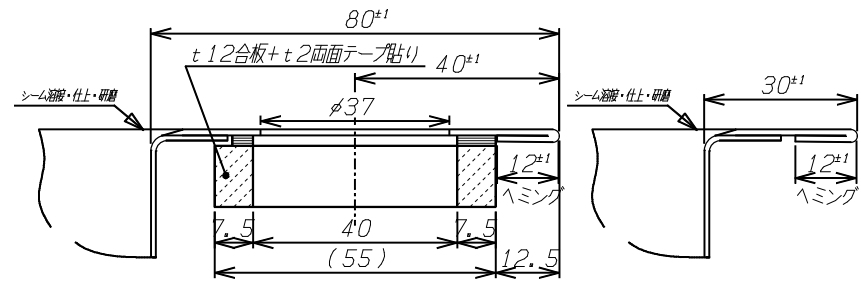
A-A' 断面 S=1/1
