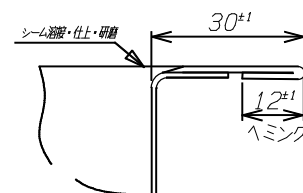
A-A' 断面 S=1/1
