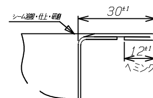
B-B' 断面 S=1/1
