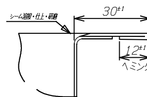
A-A' 断面 S=1/1
