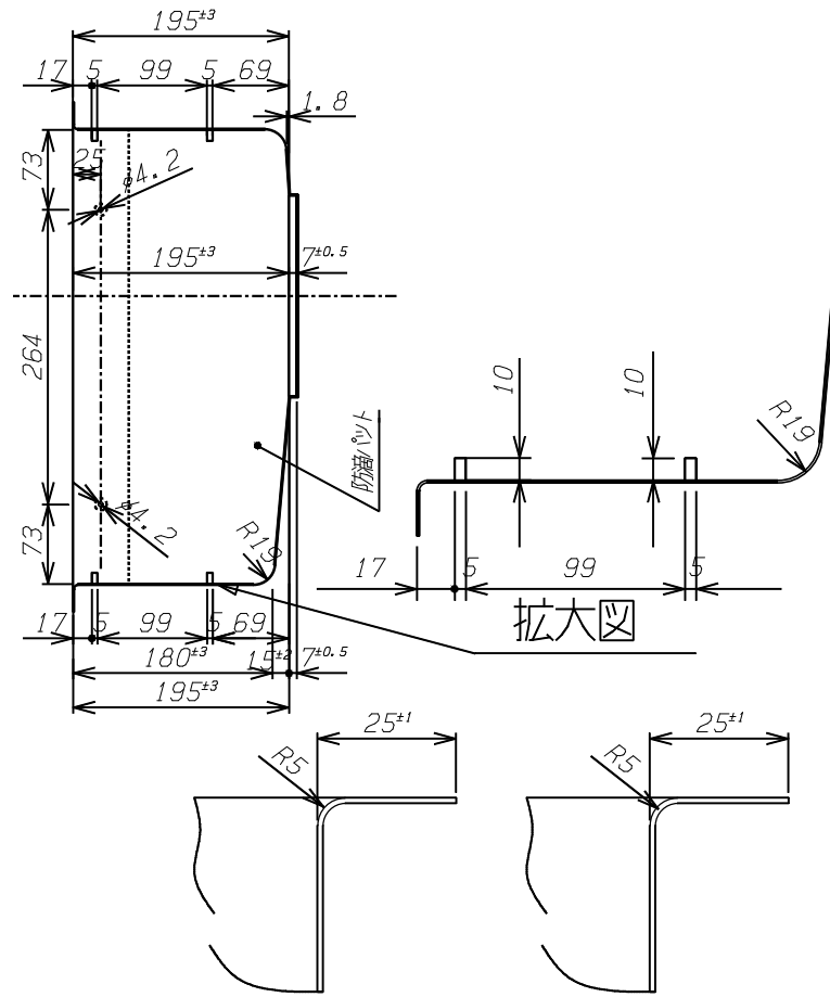
A-A' 断面 S=1/1 B-B' 断面 S=1/1
