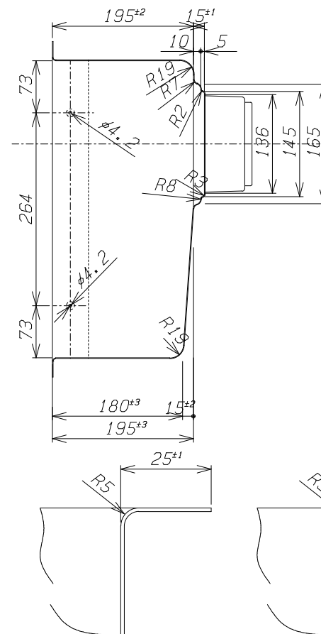
A-A' 断面 S=1/1 B-B' 断面 S=1/1
