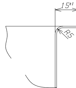
A-A断面 S=1/1
