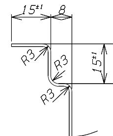
A-A' 断面S=1/1
