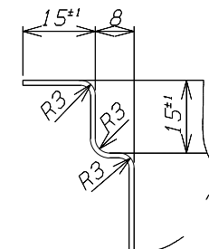
B-B' 断面S=1/1
