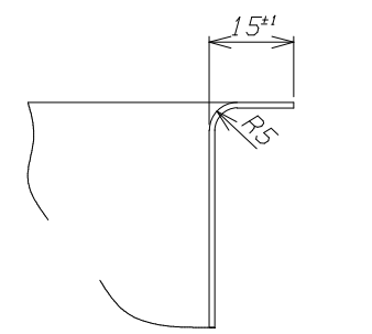
B-B' 断面 S=1/1
