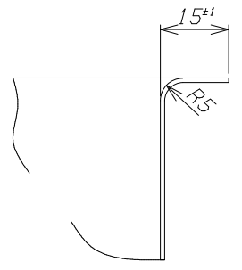
A-A' 断面 S=1/1
