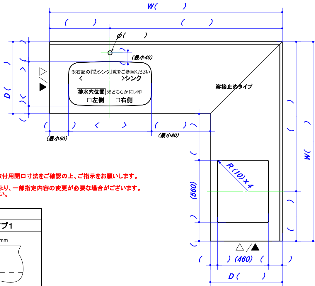
※シンク手前 最小寸法
